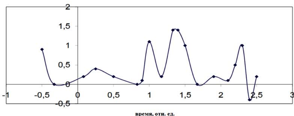
Рис. 4. Плотность тока, mA/m 2 в момент полного солнечного затмения 29 марта 2006 г. (Пролетарский пр-т, Москва): 0 – начало затмения, 14:10; 2 – конец затмения, 16:18; 1,17 – максимум затмения, 15:15, московское время [26]
