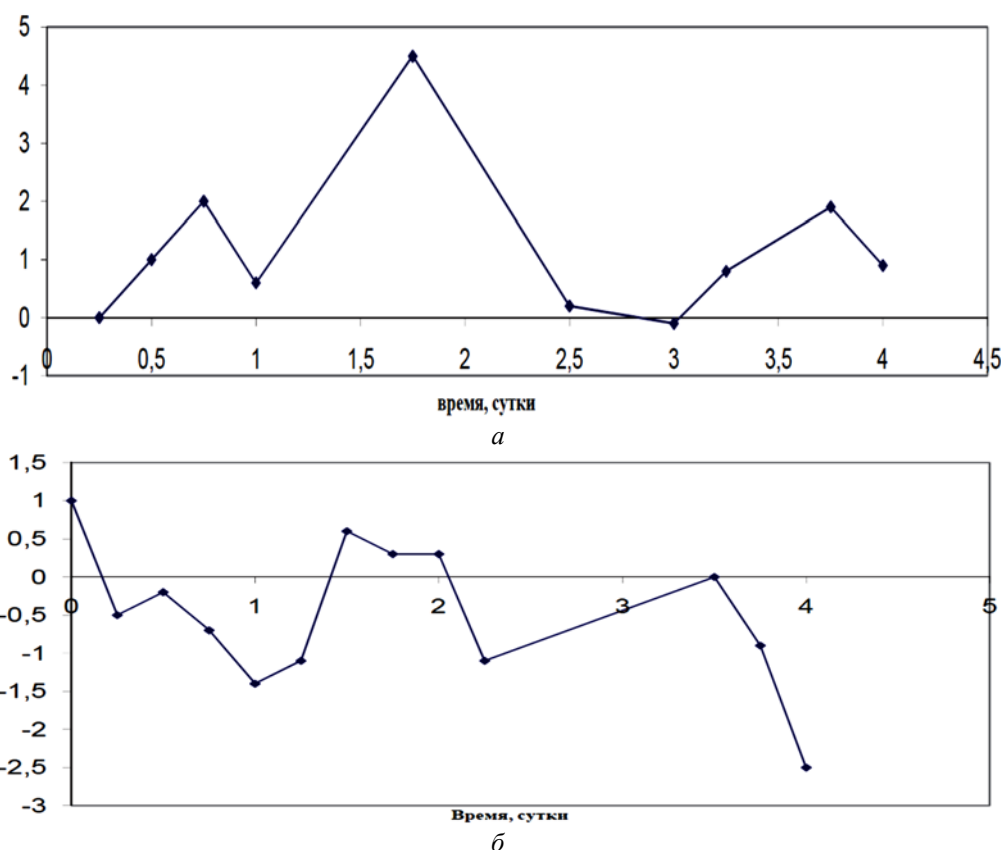
Рис. 3. Плотность вертикального тока, \text{mA}/\text{m}^2 : a – 6–9 марта 2006 г., начало отсчета – 0:00 6 марта 2006 г.; б – 13–16 марта 2006 г., начало отсчета – 0:00 13 марта 2006 г. Пролетарский пр-т, г. Москва [26]
