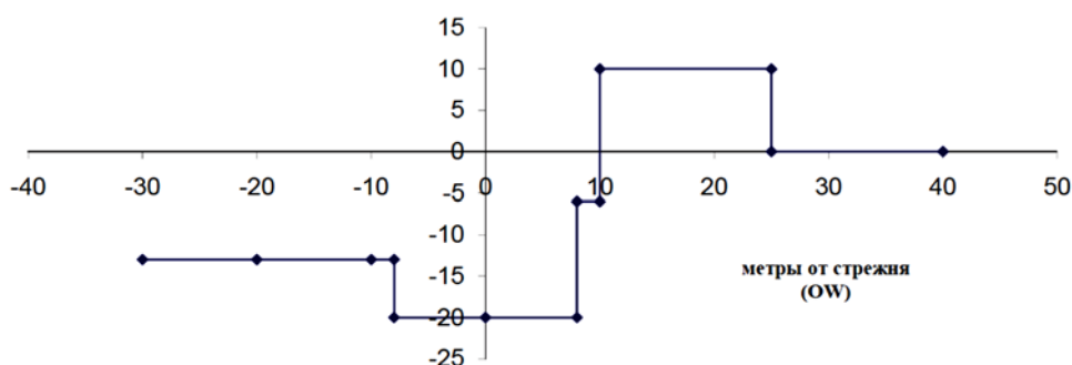
Рис. 5. Плотности тока на р. Воймега (mA/m 2 ) 24–26 августа 2006 г. [26]
