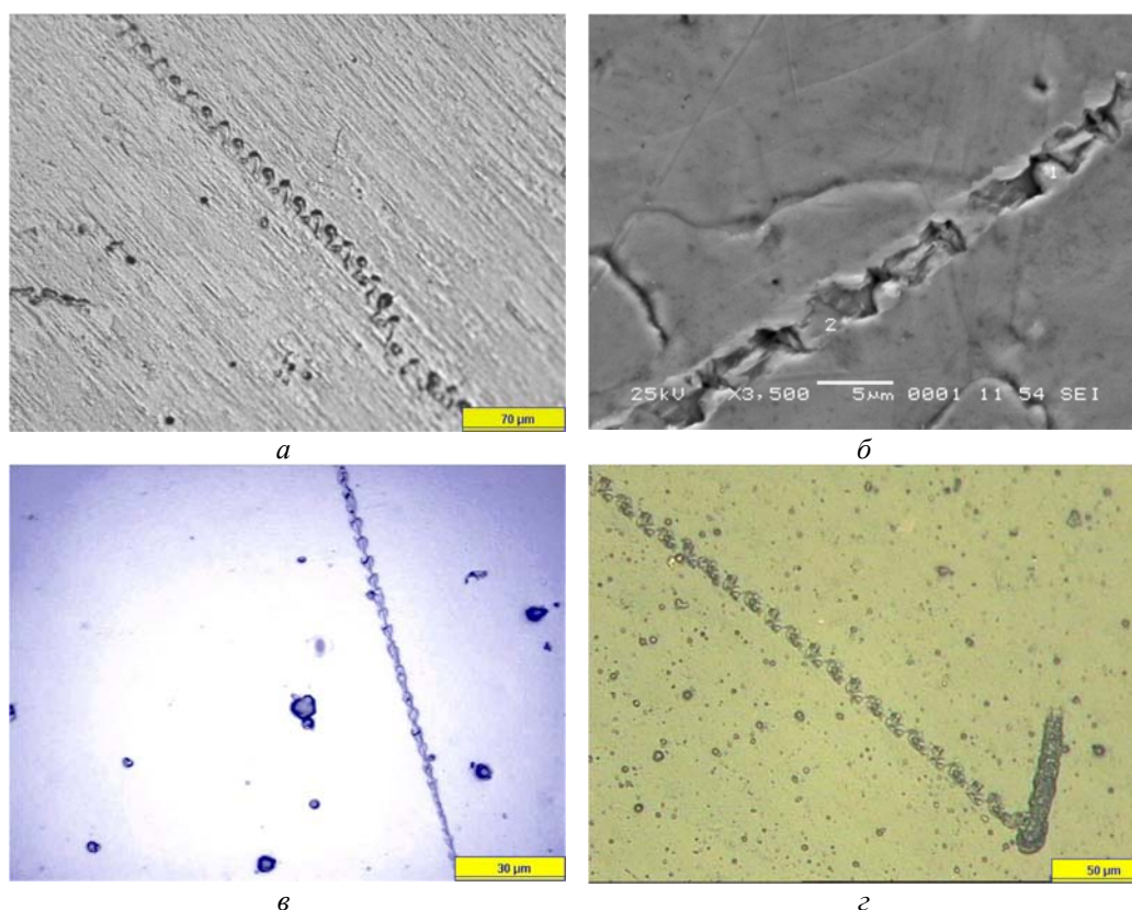
Рис. 1. Треки на поверхности палладия после облучения ионами дейтерия в тлеющем разряде: оптический микроскоп (а), электронный микроскоп (б). Примеры структур на рентгеновской плёнке, расположенной вне кварцевой разрядной камеры, после экспериментов в тлеющем разряде с цирконием (в) и палладием (г) [13]
